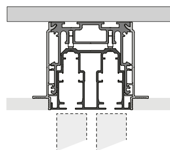
versione a soffitto (B) ceiling version (B)
