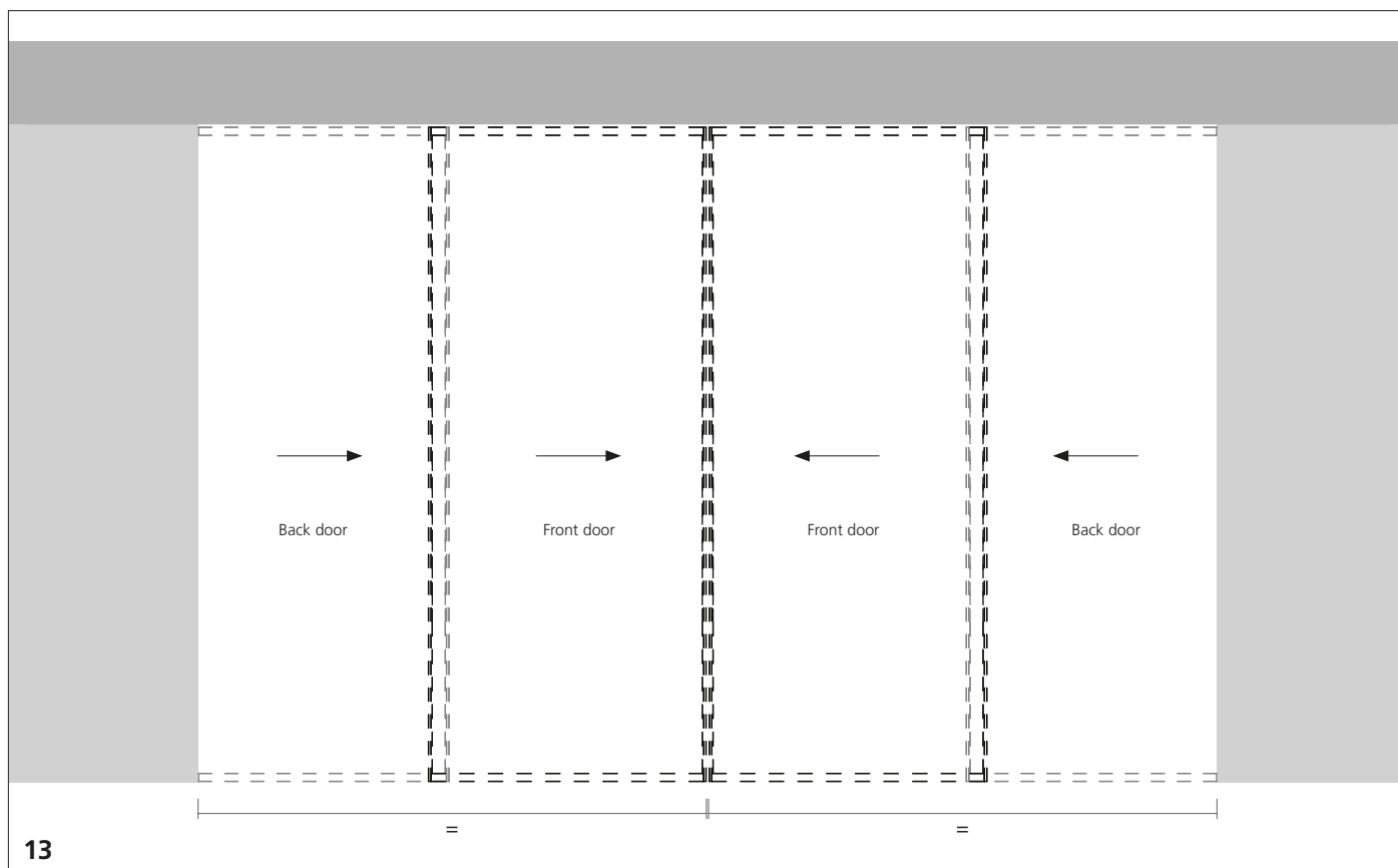
13. Installare le ante come descritto nelle pagine da 2.2.227 a 2.2.233. Verificare la perfetta chiusura delle ante nella mezzera del vano. 13. Install the doors as shown on pages from 2.2.227 to 2.2.233. Check the perfect closure of the doors in the opening centerline.
