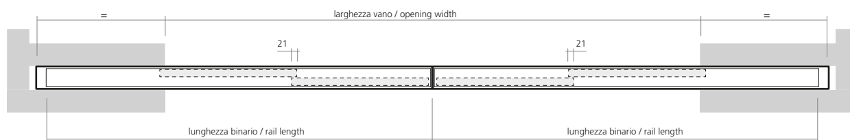
versione a soffitto (B) ceiling version (B)
